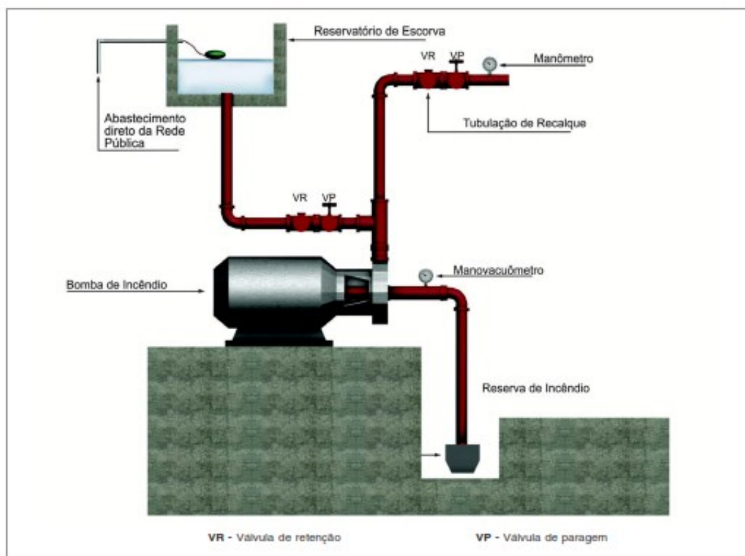
Figura C.3: Exemplo de afogamento de bomba de incêndio
