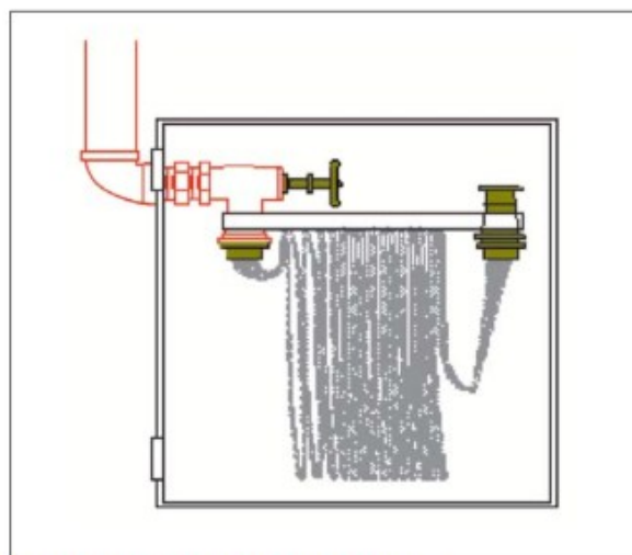
Figura 3: Suporte para mangueira tipo "rack"
