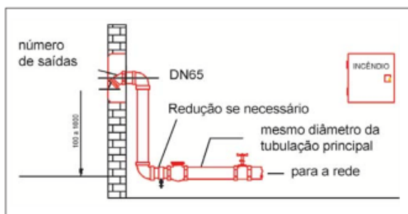
Figura 1: Dispositivo de recalque tipo coluna
